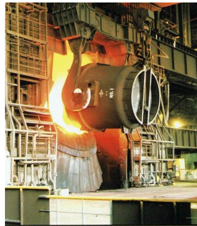
転炉
