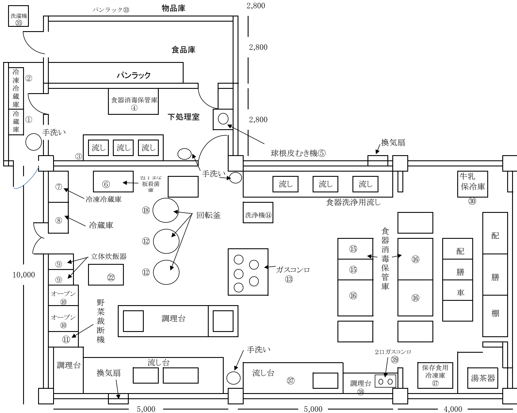
向日が丘支援学校 厨房機器現況図
