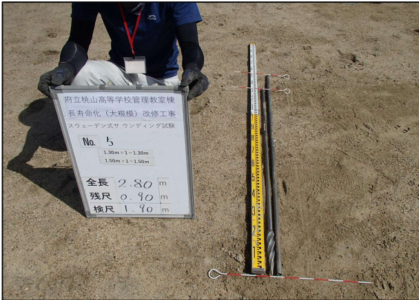
No.5 検尺
