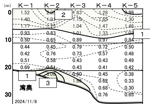
栗田湾 11月 蛍光量
