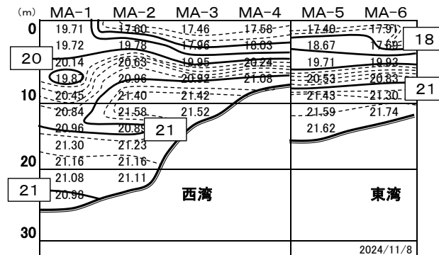
舞鶴湾 11月 塩分
