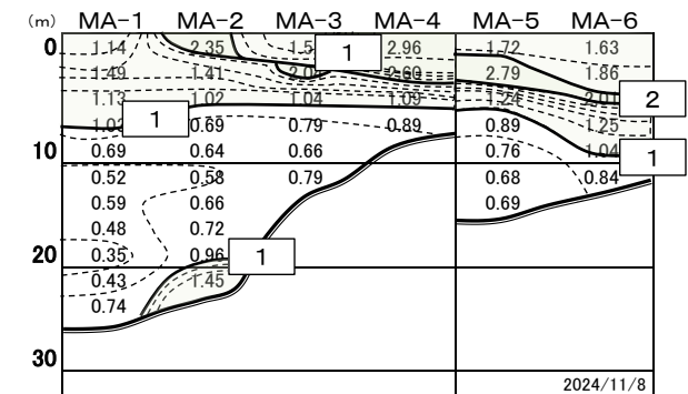
舞鶴湾 11月 蛍光量
