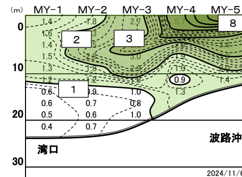
宮津湾 11月 蛍光量
