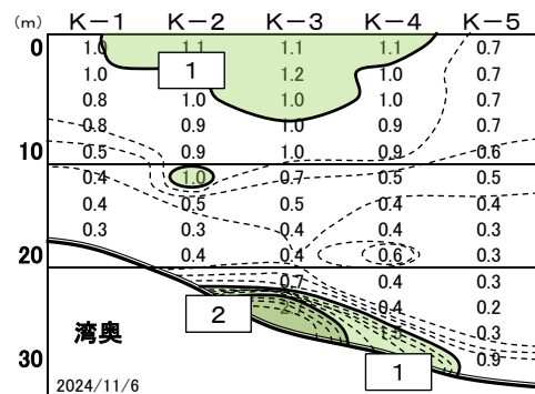
栗田湾 11月 蛍光量
