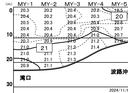
宮津湾 11月 塩分
