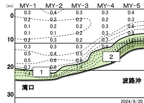
宮津湾 9月 蛍光量
