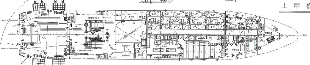
上甲板下
