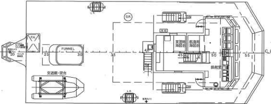
航海船橋甲板
