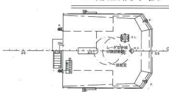
上部船橋甲板
