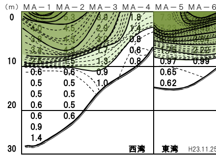
舞鶴湾 2011年(平成23年)11月 蛍光量
