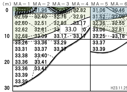
舞鶴湾 2011年(平成23年)11月 塩分濃度
