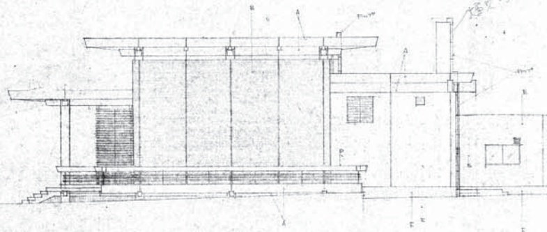
東側立面圖
