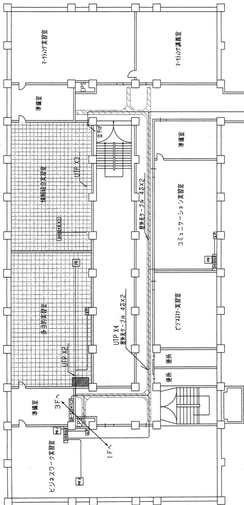
資料 4-13 京都すばる高等学校生徒用 LAN 配線図（実習棟 2 階）
