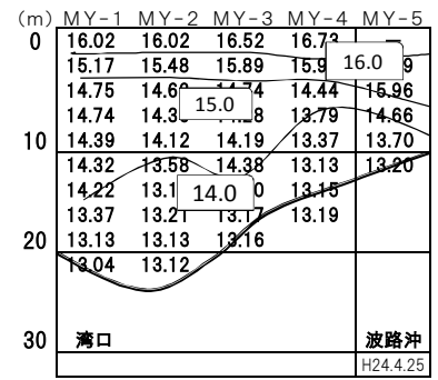
宮津湾 2012年(平成24年)4月 塩分濃度
