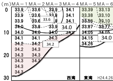
舞鶴湾 2012年(平成24年)4月 塩分濃度
