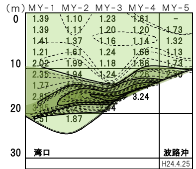
宮津湾 2012年(平成24年)4月 蛍光量
