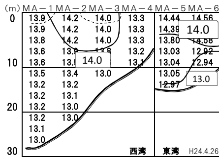
舞鶴湾 2012年(平成24年)4月 水温
