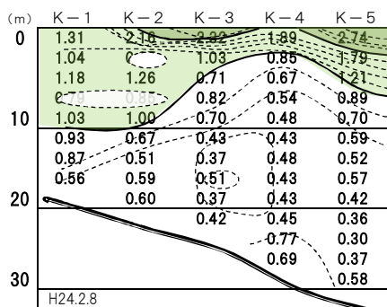
栗田湾 2012年(平成24年)2月 蛍光量
