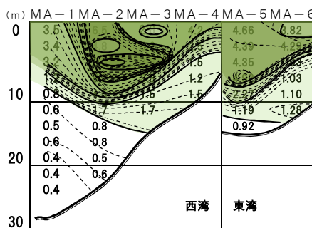
舞鶴湾 2012年(平成24年)2月 蛍光量
