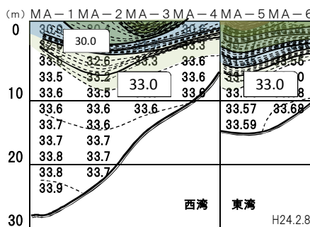
舞鶴湾 2012年(平成24年)2月 塩分濃度
