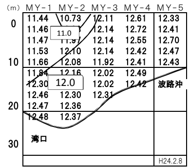
宮津湾 2012年(平成24年)2月 水温
