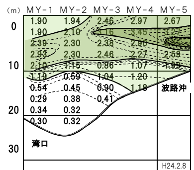
宮津湾 2012年(平成24年)2月 蛍光量
