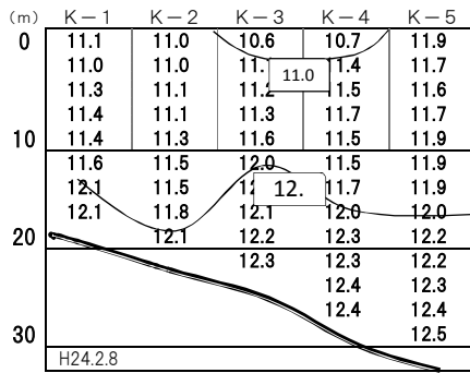
栗田湾 2012年(平成24年)2月 水温
