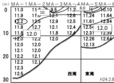
舞鶴湾 2012年(平成24年)2月 水温
